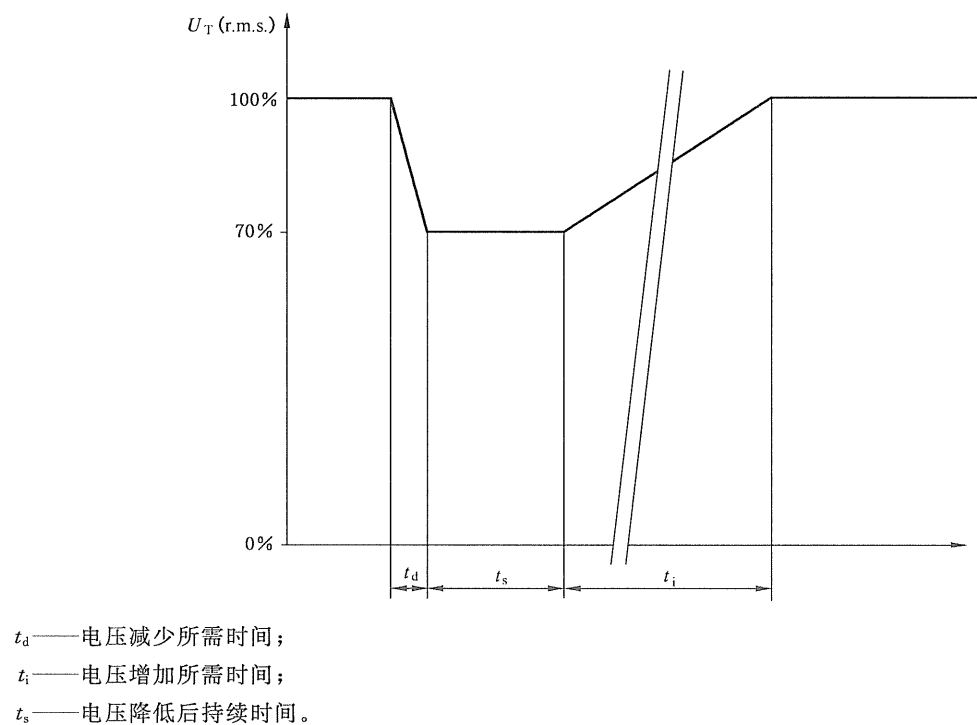
图 3 电压变化
